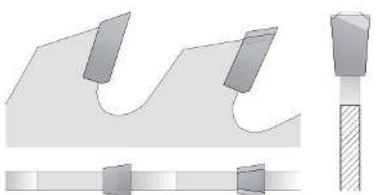
Трапецевидный плоский зуб
