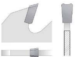
Заточка «Дупловит» с фаской
