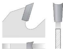
Заточка «Дупловит» полый торец
